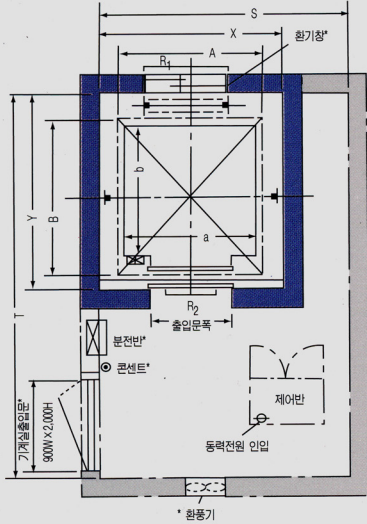
승강로 및 기계실 평면도(1대 단독)
