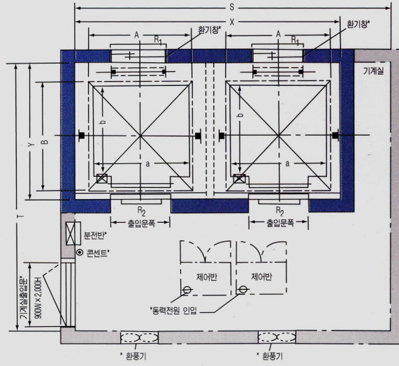
승강로 및 기계실 평면도(2대 병렬)
