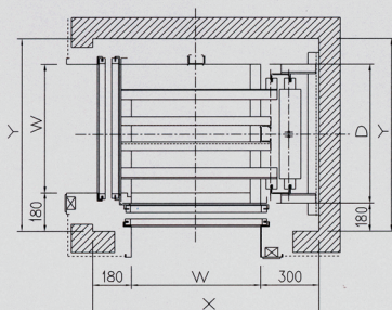
• C-TYPE : 직각관통형
