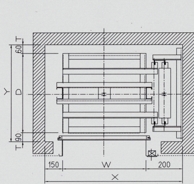
• A-TYPE : 일방형 (관통형일 경우 T:130)
