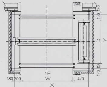
• D-TYPE : 관통형(급식용)
