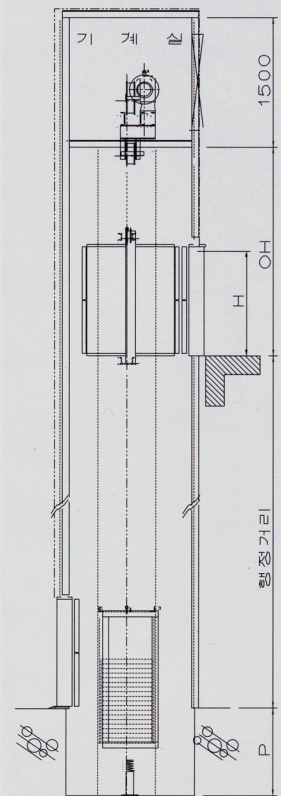
● 플로어 타입 단면도
