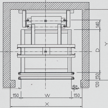
• B-TYPE : 일방형(카도어)
